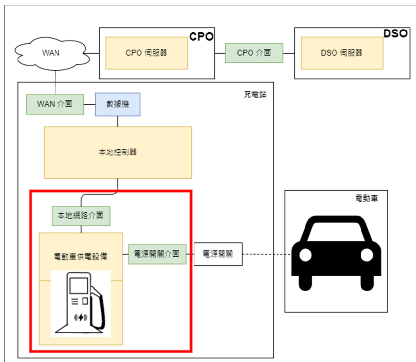
圖 1 電動車供電系統基本架構示意圖
